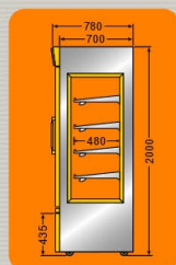
CR-MD1825 六尺開門式蛋糕展示櫃
