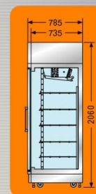
TB-U720S 機組上置型冷凍冷藏櫃
