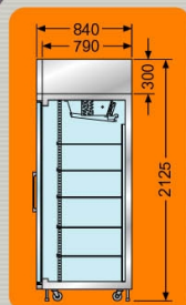
AT-R11420S 二門機組上置型冷凍冷藏櫃
