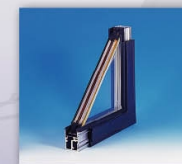
◎門框鋁料厚實、抗拉強度佳。門框迫緊膠條吸附面寬闊、密閉性強、冷氣不外漏。複層式防霧玻璃厚度達28mm、保冷、省電。
